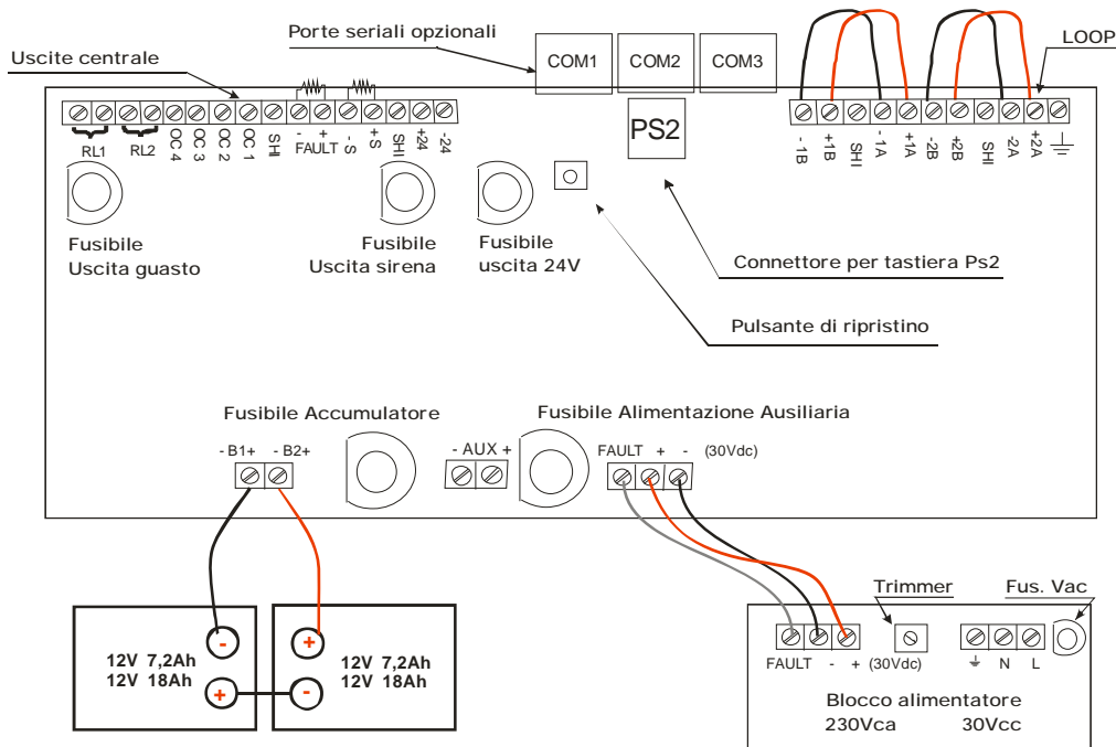
Fig. 2 – Descrizione della scheda elettronica della centrale.
